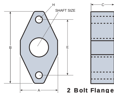
2 Bolt Flange
